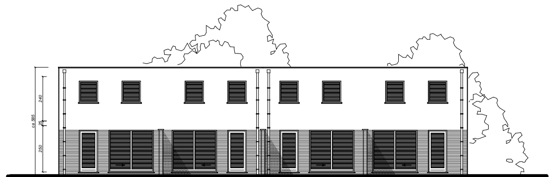
achtergevel
